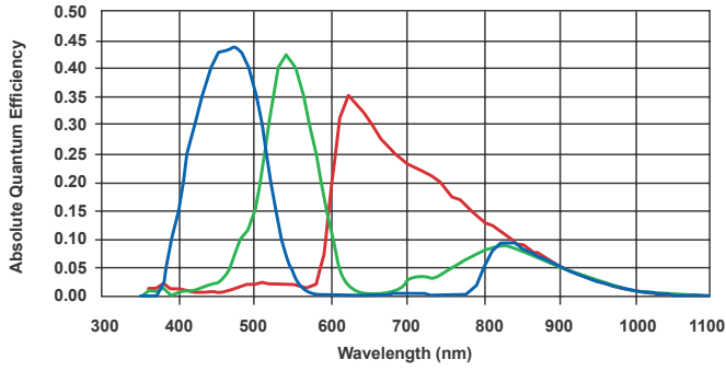
TMC-6740 1/3" 640 (H) x 480 (V) KAI-0340
