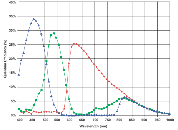
TMC-1000 1" 1024 (H) x 1024 (V) KAI-1010 TMC-1020 1" 1024 (H) x 1024 (V) KAI-1010
