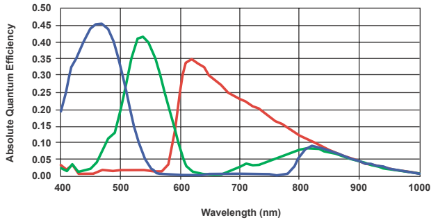
TMC-4100 1.2" 2048 (H) x 2048 (V) KAI-4021
